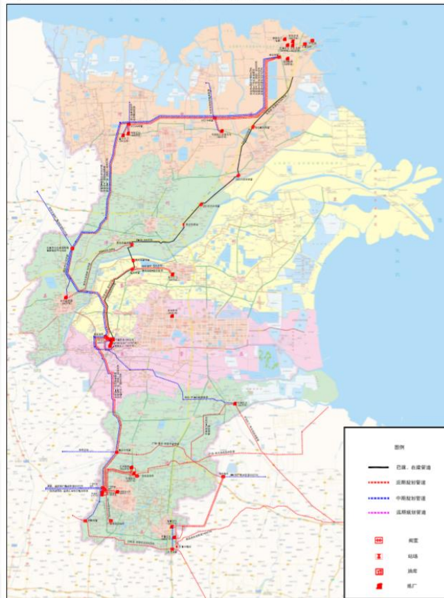
附图3 东营市成品油管网建设规划图
